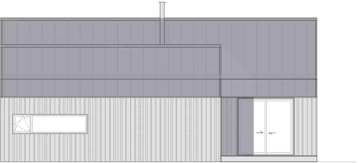
ZÁPADNÍ POHLED
