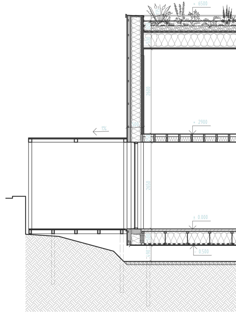
Čiastkový rez domom
