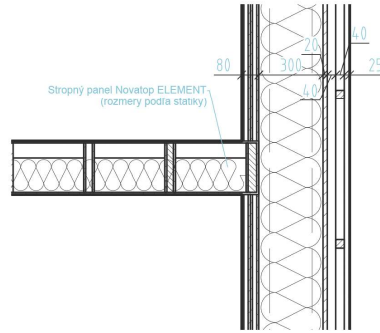
Detail napojenia stropnej konštrukcie na obvodovú stenu
