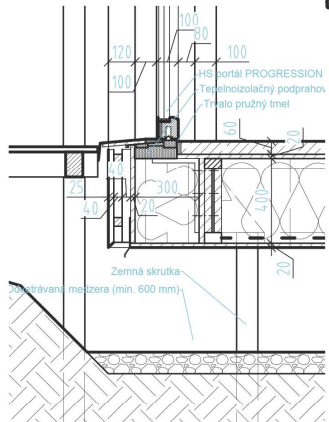
Detail výstupu na terasu
