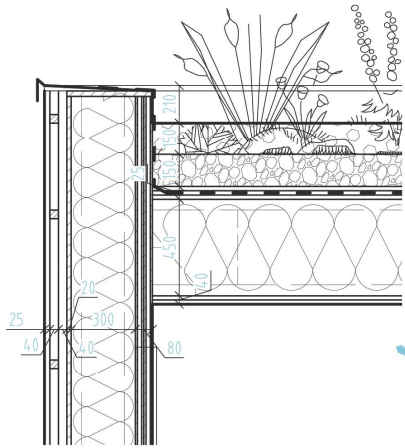
Detail strešnej konštrukcie pri atike
