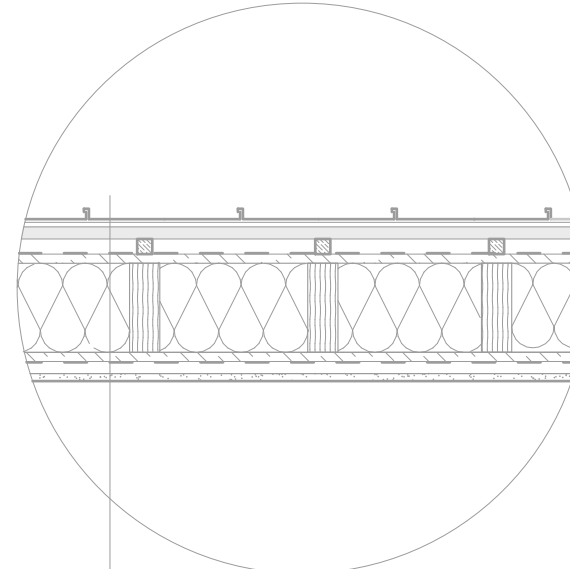
SKLADBA STRECHY
