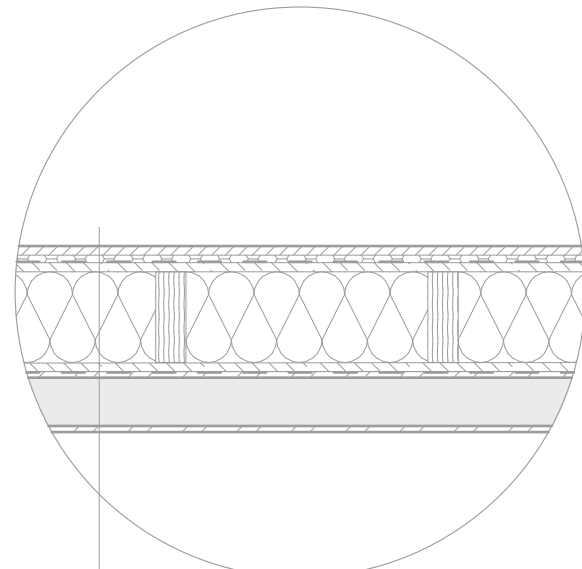
SKLADBA PODLAHY
